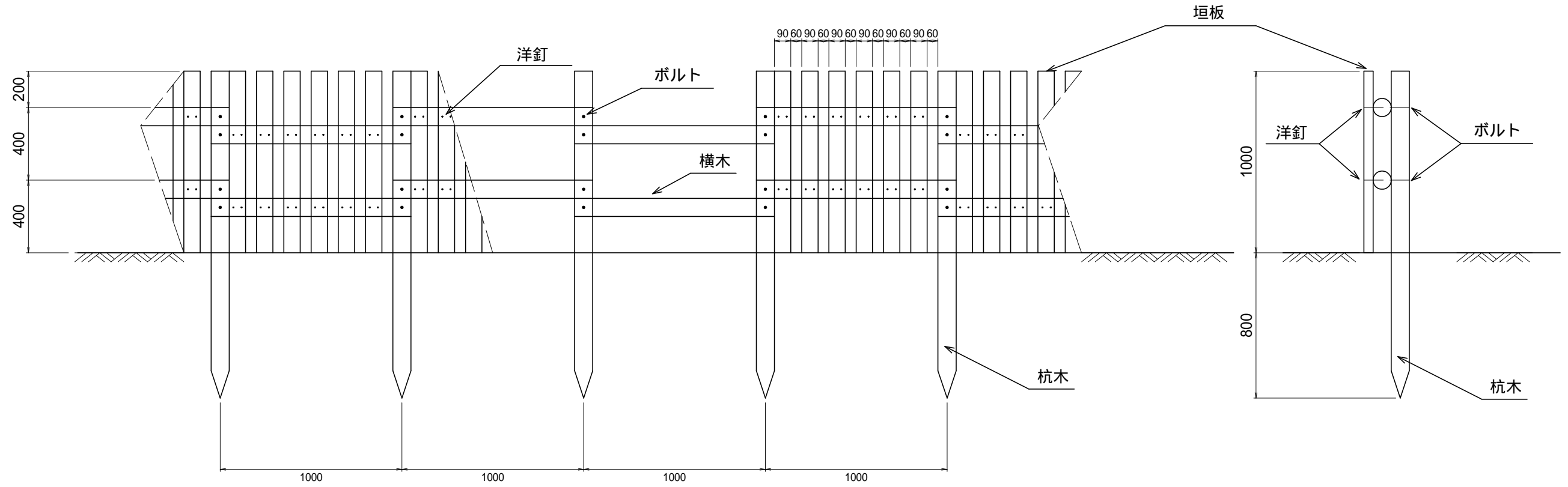
正面図
